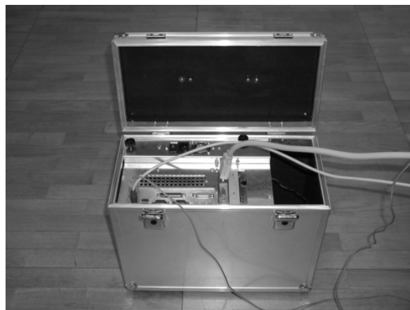
Bild 2. Mobiler PC mit Dualhead-Graphikkarte.
